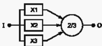
Рисунок 6 — Резервирование 2/3
