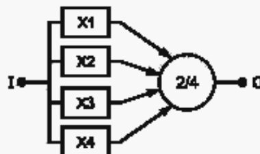
Рисунок 7 — Резервирование 2/4
